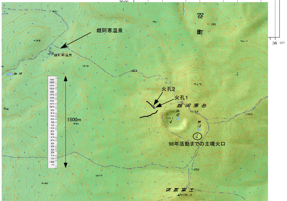
図2. ヘリコプター観測によって確認された火口位置図(札幌管区気象台提供資料に加筆修正)
