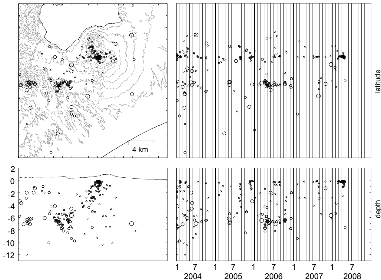
図1. 北海道大学の火山観測網で検知された樽前山周辺の地震活動
