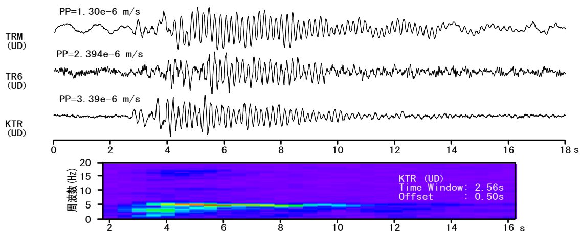
図2. TRM, TRG, KTRで観測された単色地震(上下動成分)とランニングスペクトル(KTR)
