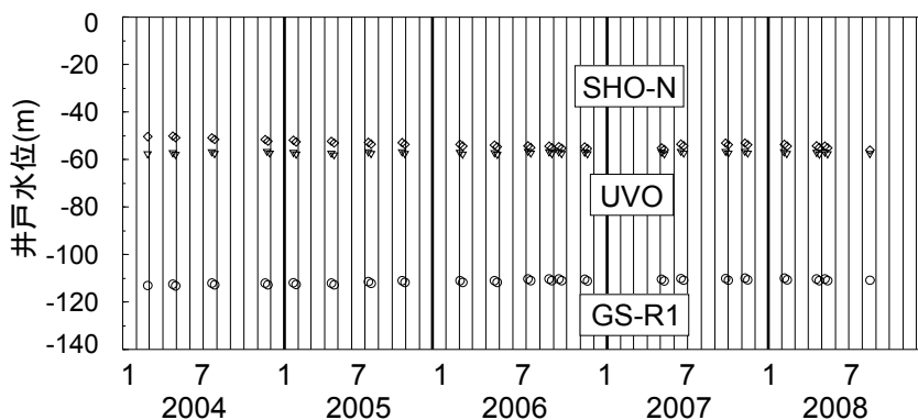
図2. 昭和新山周辺の井戸水位変化
