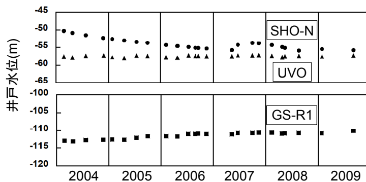
図2. 昭和新山周辺の井戸水位変化
