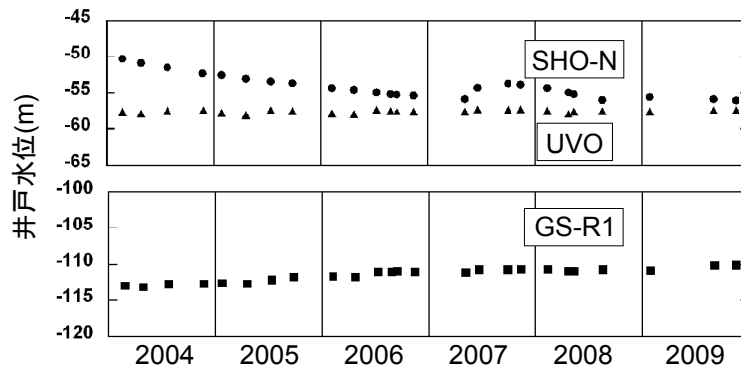
図2. 昭和新山周辺の井戸水位変化
