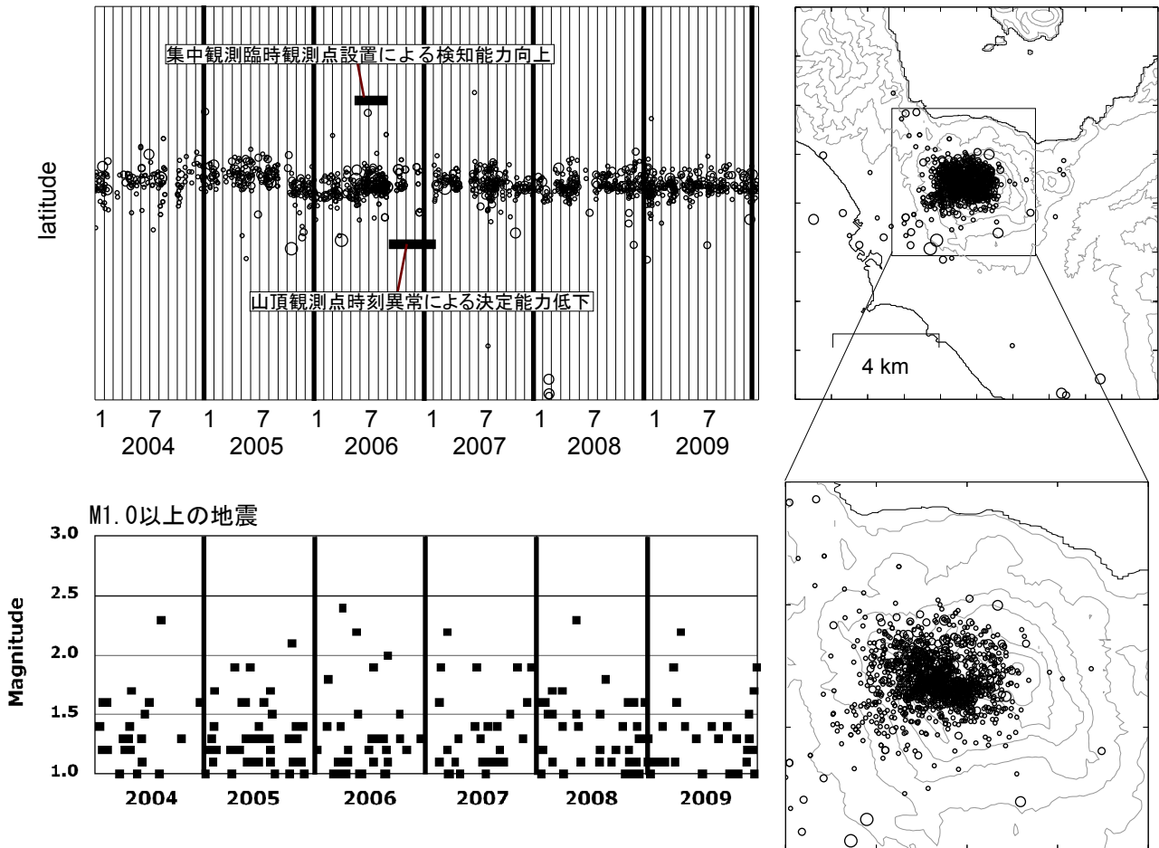
図1. 北海道大学の火山観測網で検知された有珠山周辺の地震活動
