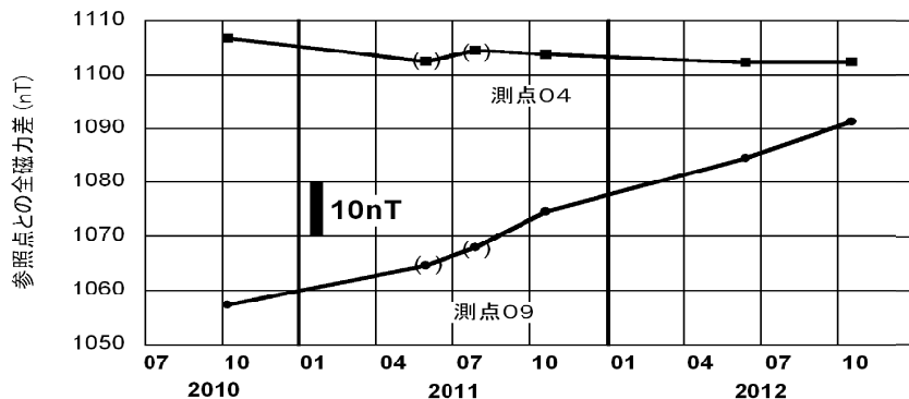
図2. 測点04と09の全磁力変化時系列(参照点は00地点。括弧付きは参考値)
